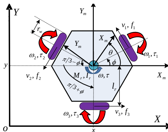
萬向輪機器人之軌跡追蹤
