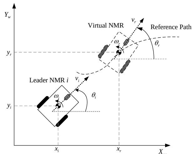
多機器人之隊形控制
