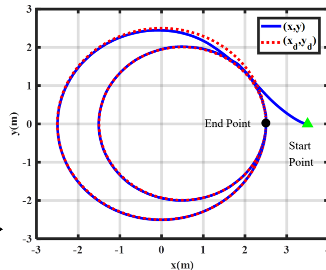
萬向輪機器人之軌跡追蹤
